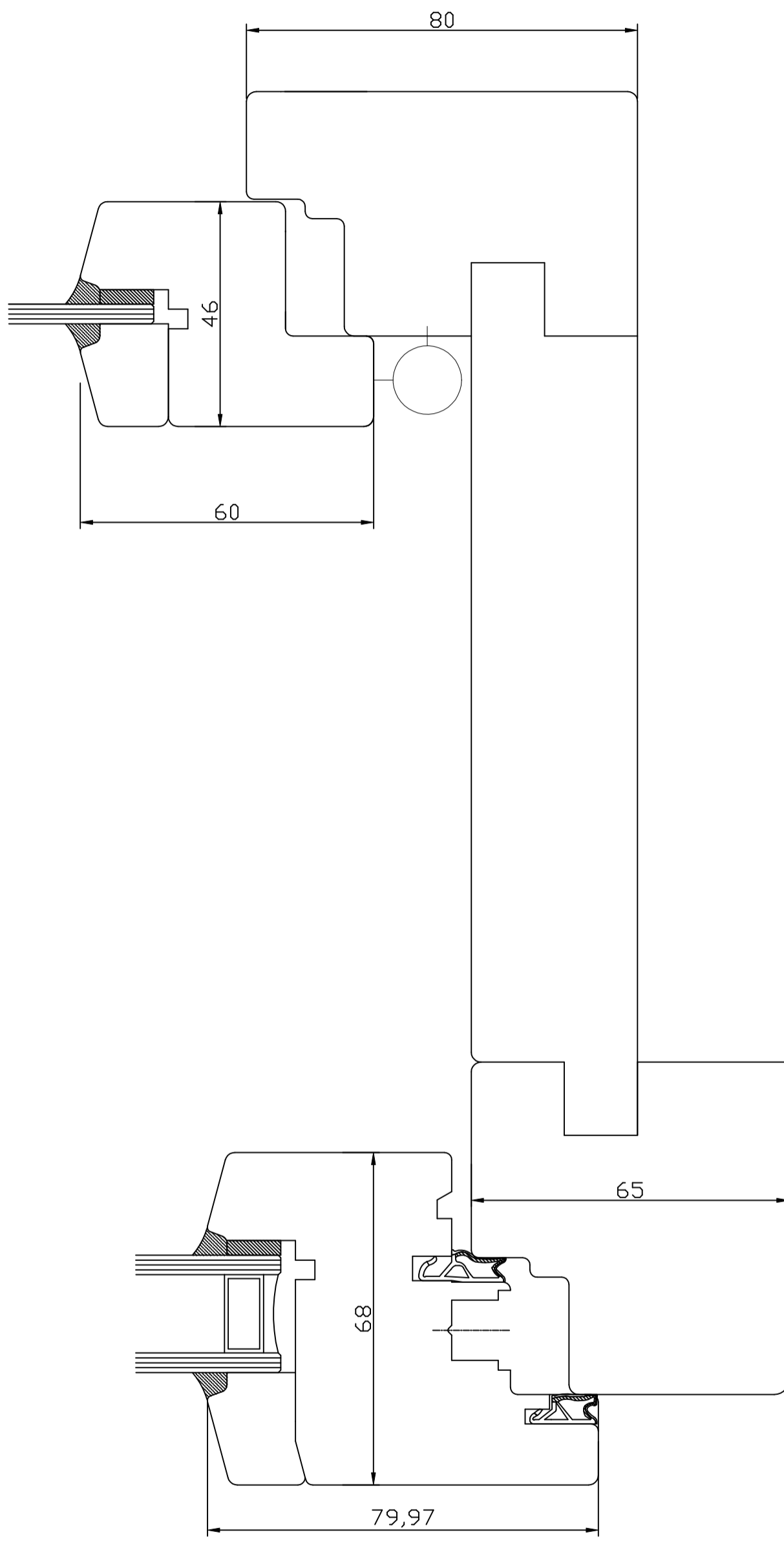
Stojak okna skrzynkowego
